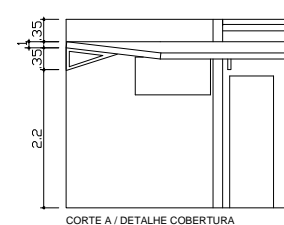
CORTE A / DETALHE COBERTURA TEL. A ISOTÉRMICA sem escala
