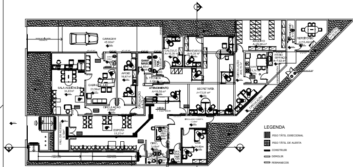
V.T. CERES PLANTA BAIXA LAYOUT Esc: 1/100
