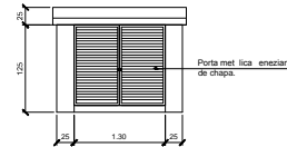
VISTA FRONTAL sem escala
