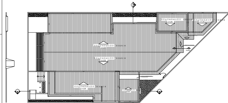
V.T. CERES PLANTA DE COBERTURA Esc: 1/100
