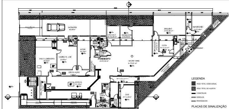
V.T. CERES PLANTA BAIXA / LOCAÇÃO Esc: 1/100
