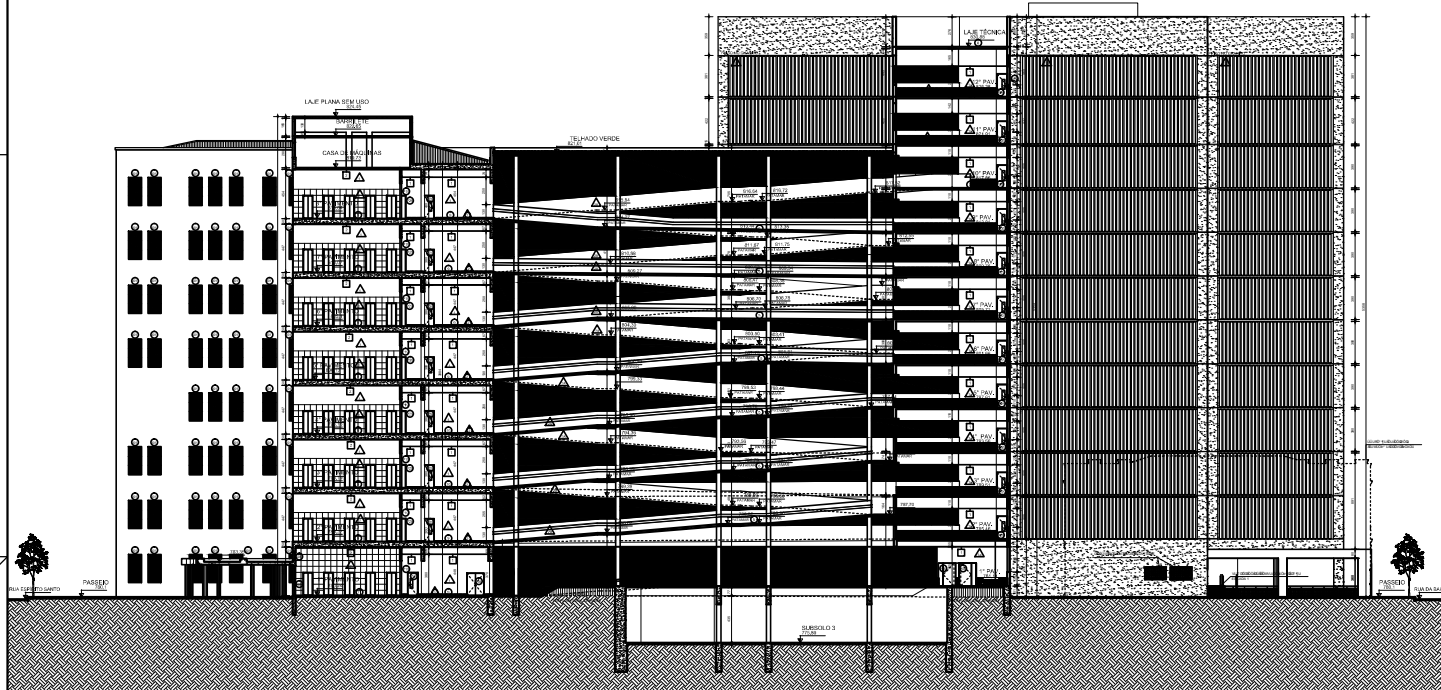
CORTE AA
