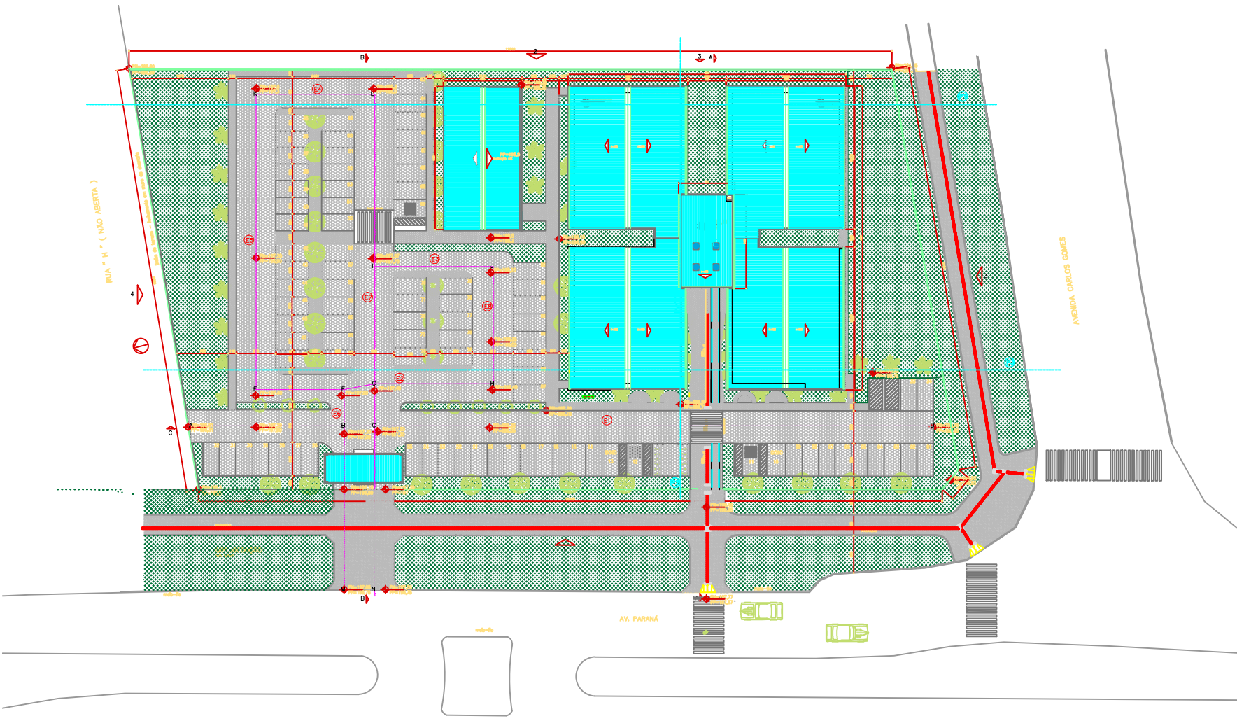
IMPLANTAÇÃO ESC 1:1000
