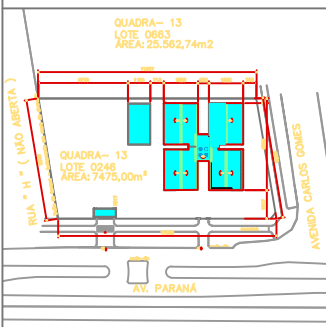
SITUAÇÃO ESC 1:1000
