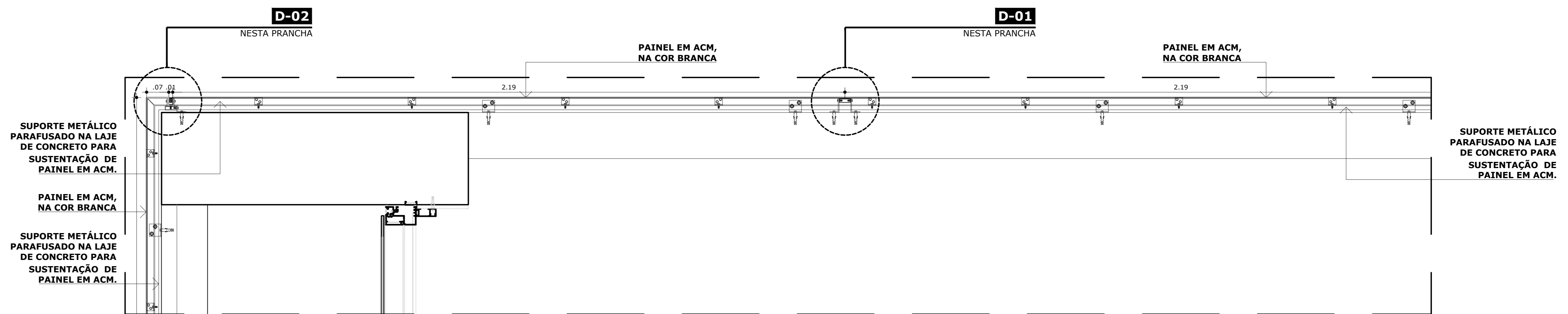
07 PL. BAIXA FRONTÃO - MÓDULAÇÃO ACM ESCALA 1/10
