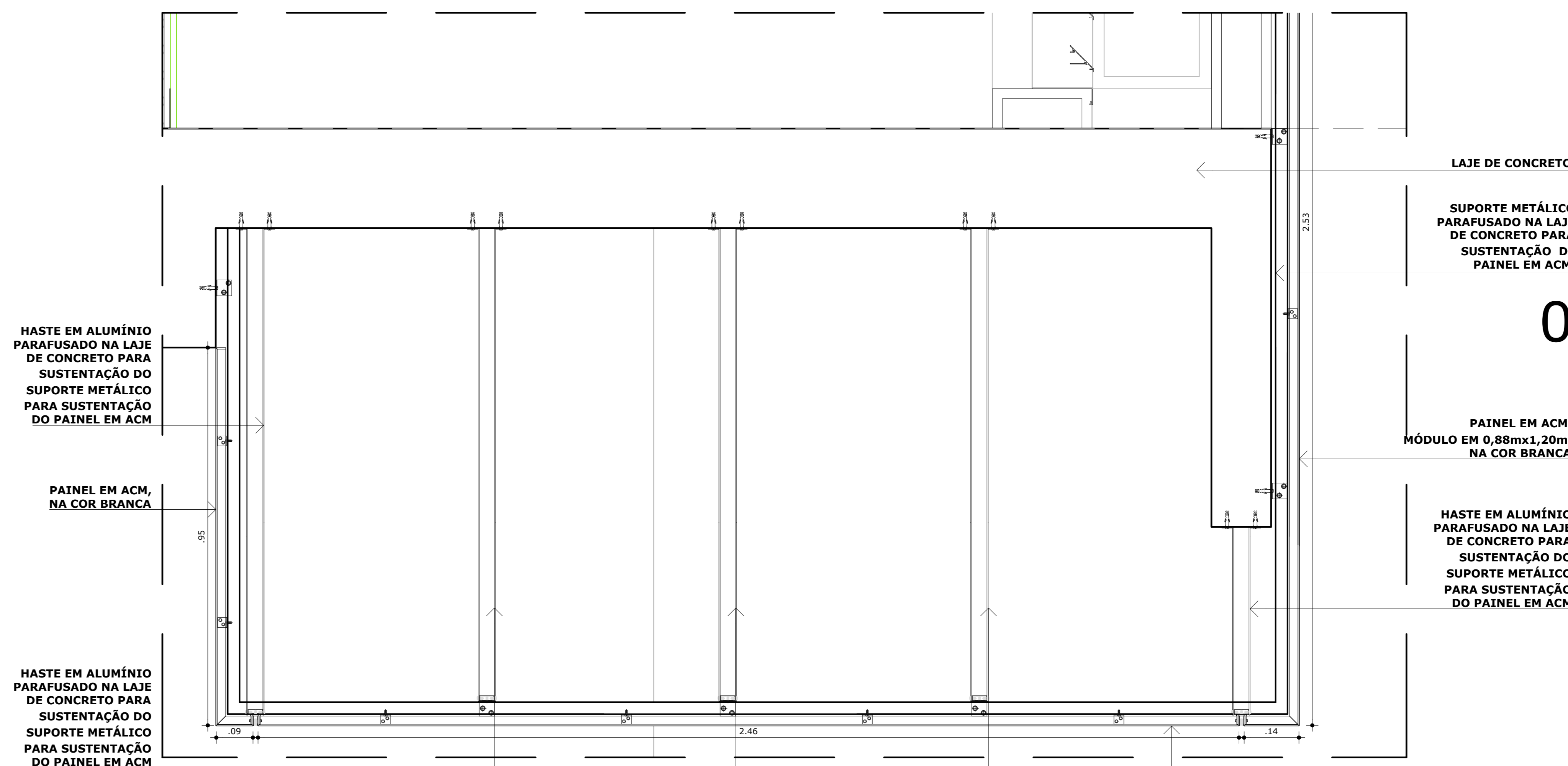
06 DET. 04 - FIXAÇÃO ACM INFERIOR ESCALA 1/10
