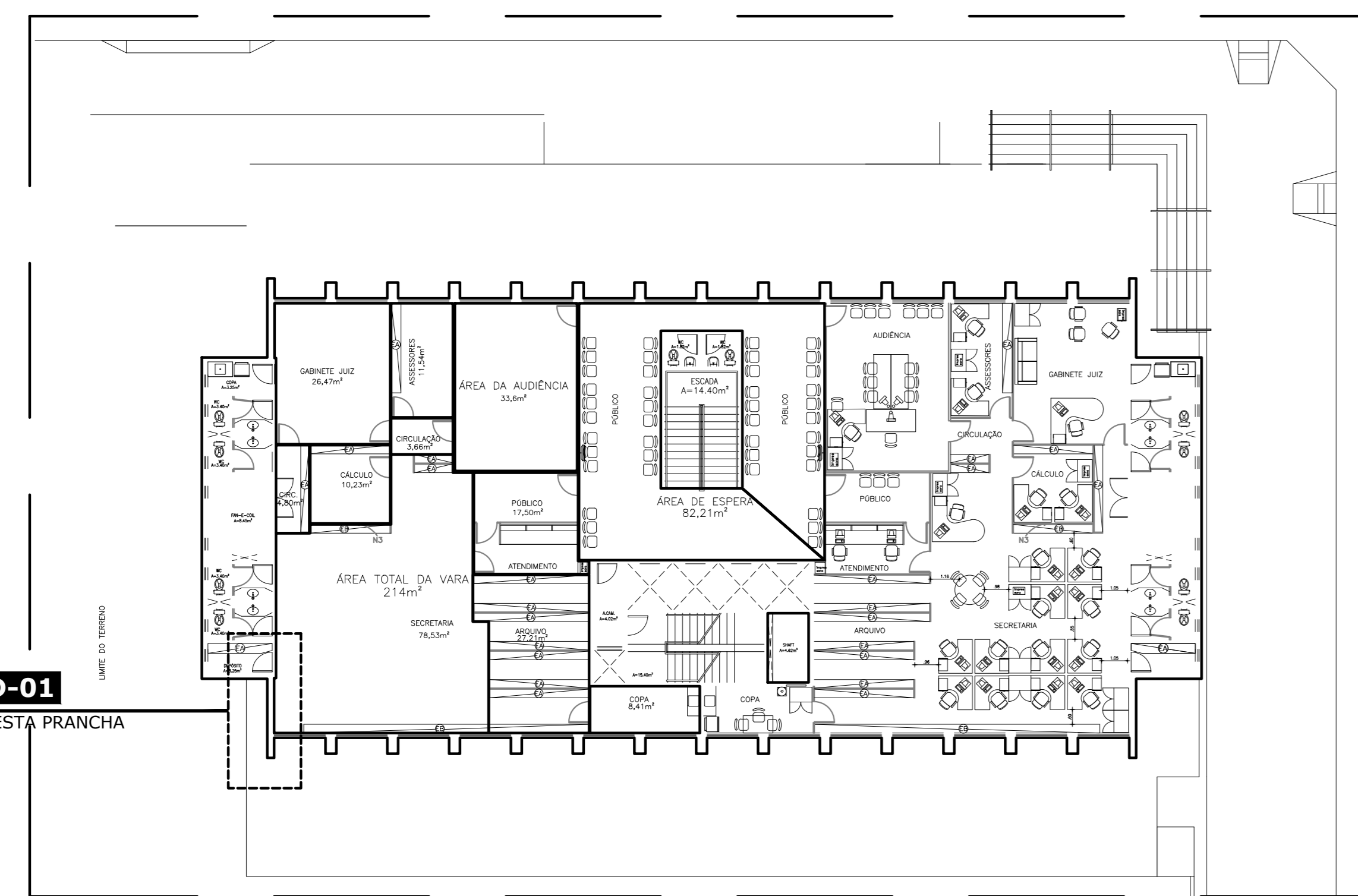
01 PL. LOCALIZAÇÃO ACM ESCALA 1/250
