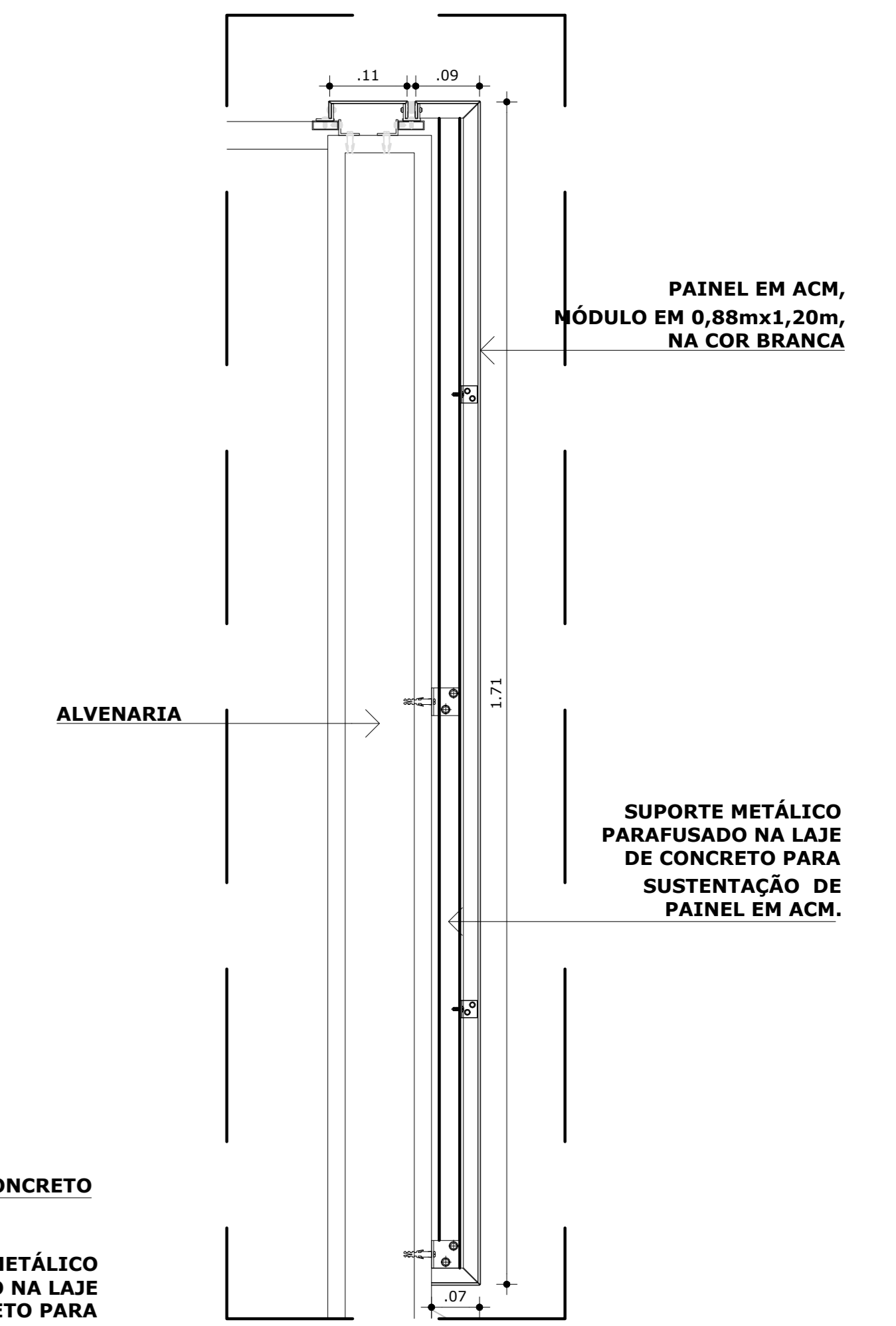
05 DET. 03 - FIX. ACM SUPERIOR ESCALA 1/20
