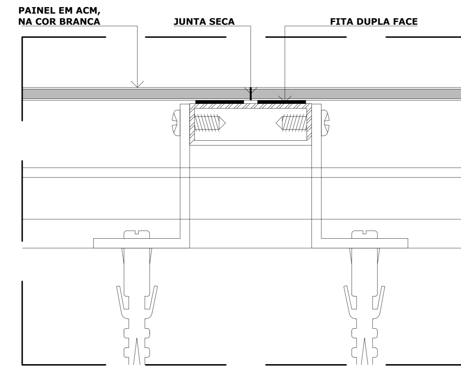
03 DET. 01 - JUNTA SECA ESCALA 1/1
