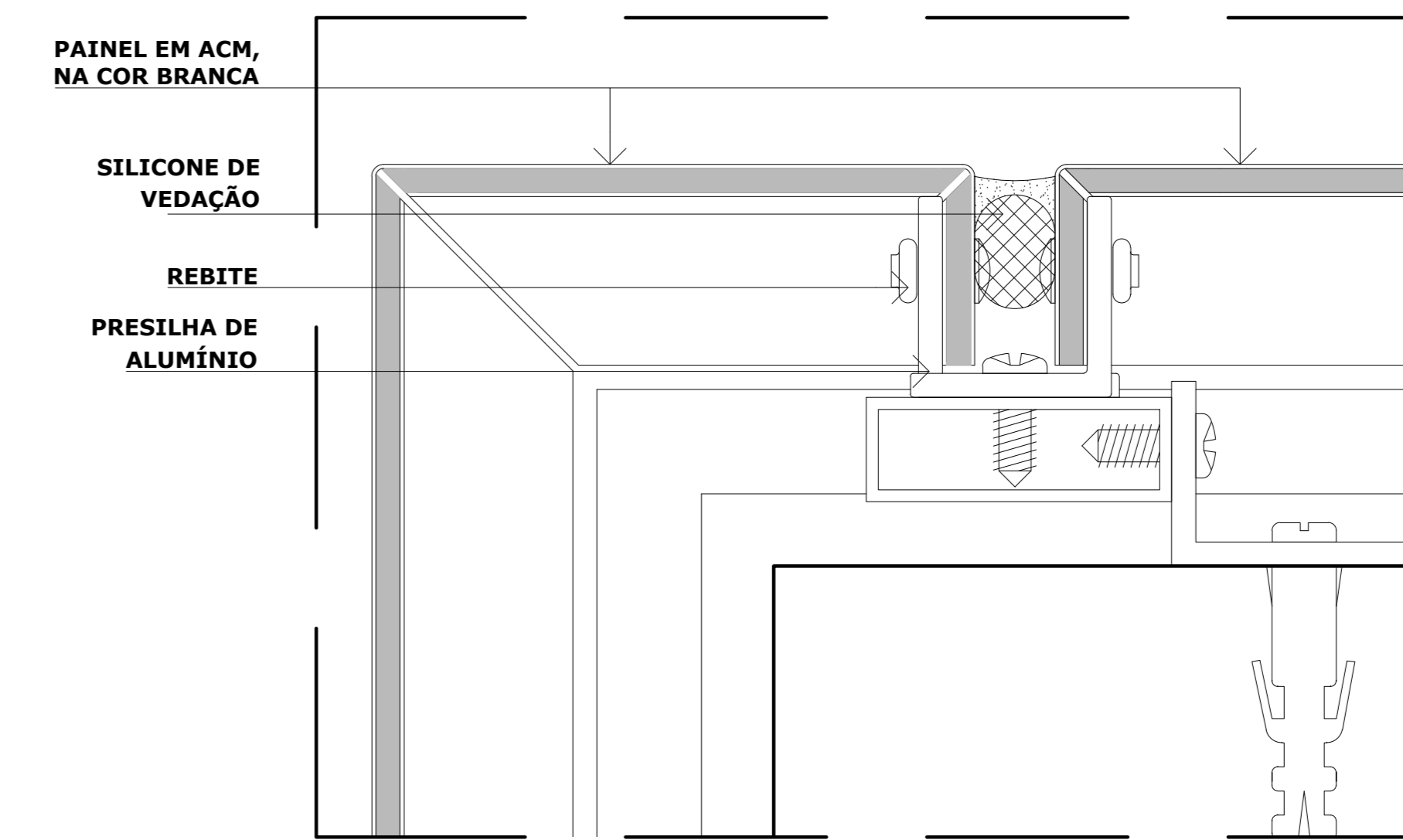
04 DET. 02 - DET. DE CANTO ESCALA 1/1
