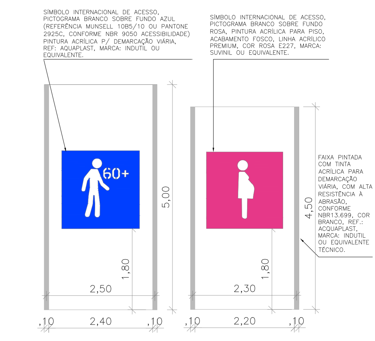
02 - DET. VAGAS ESPECIAIS ESCALA: 1/50
