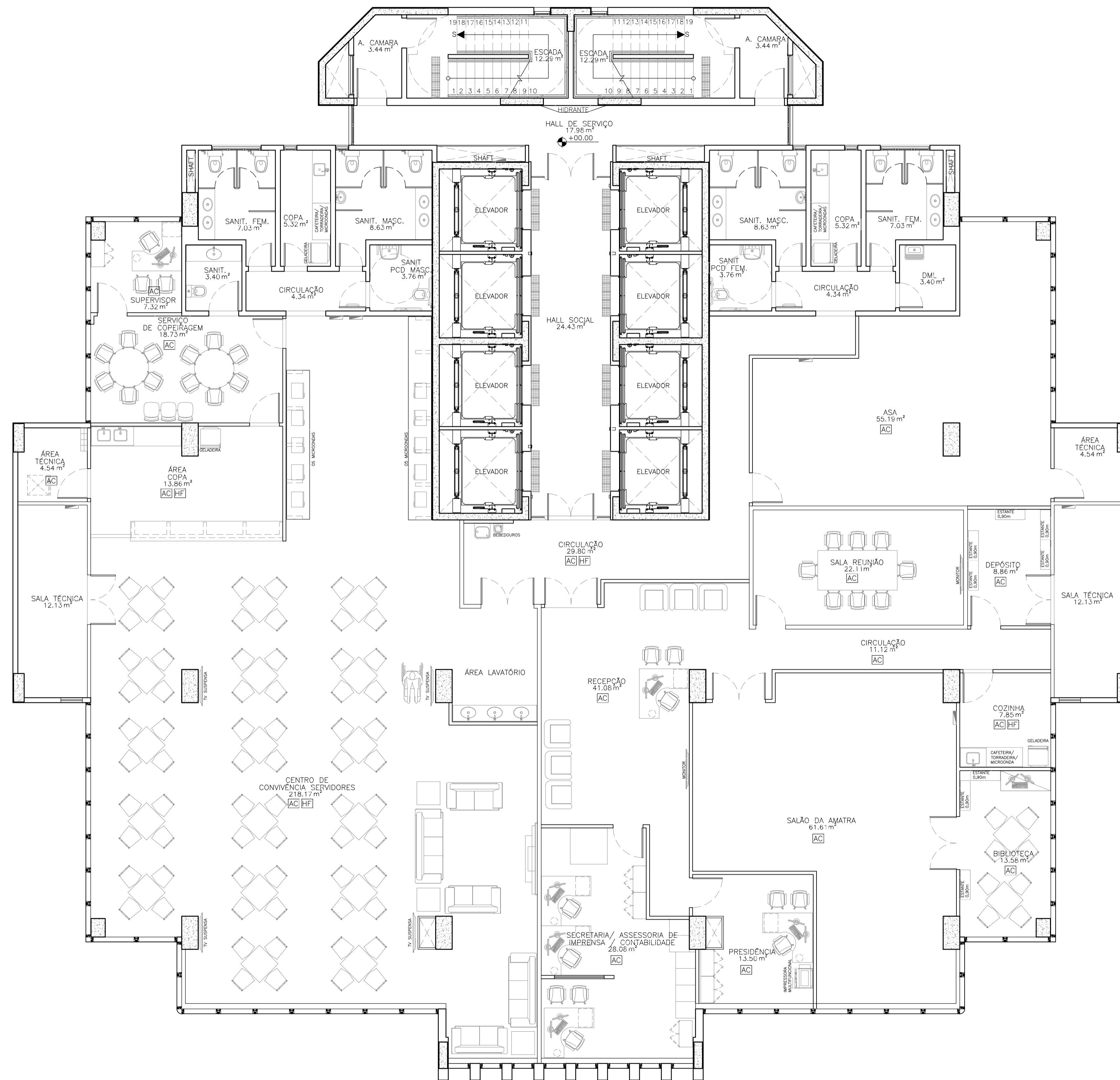
01 PLANTA LAYOUT – 10º PAV. ESCALA: 1/75
