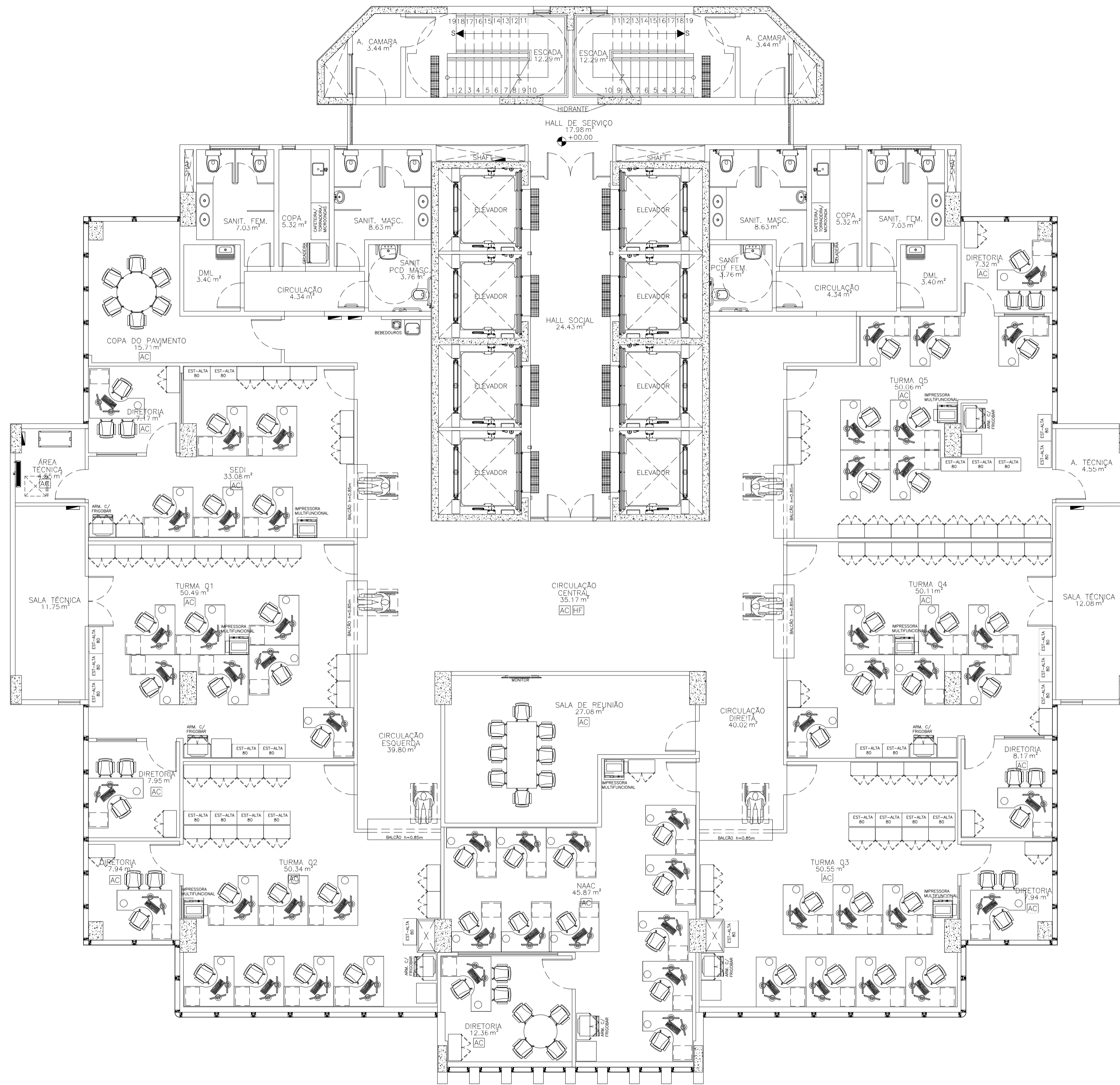
01 PLANTA LAYOUT – 4º PAV. ESCALA: 1/75
