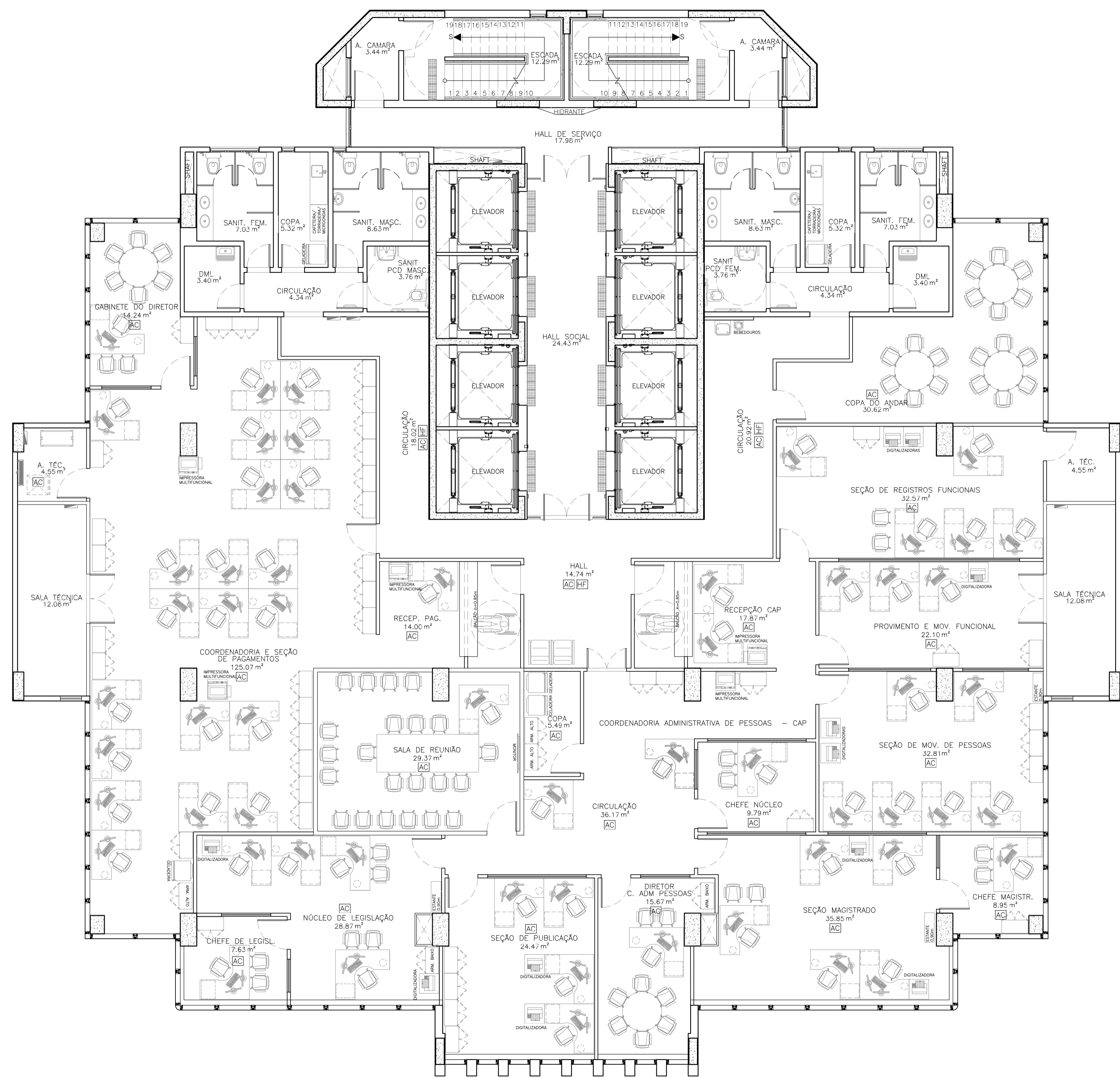
01 PLANTA LAYOUT – 6º PAV. ESCALA: 1/75
