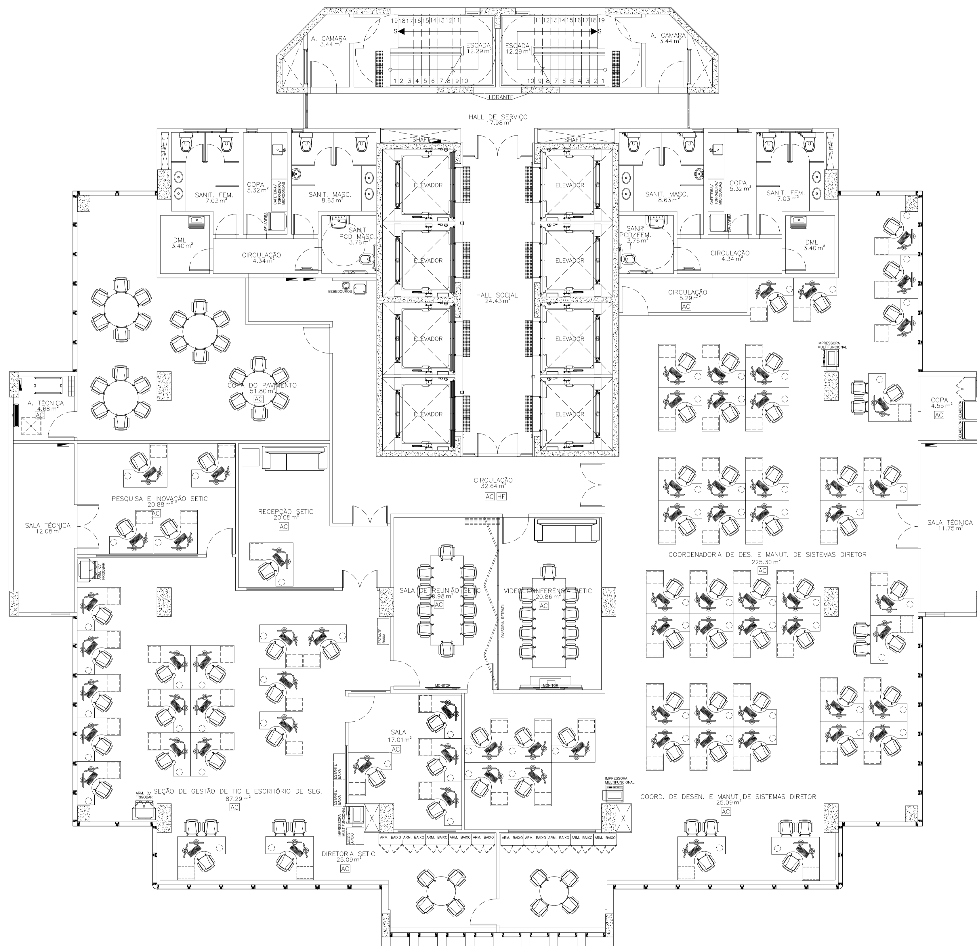
01 PLANTA LAYOUT – 1º PAV. – ESCALA: 1/75
