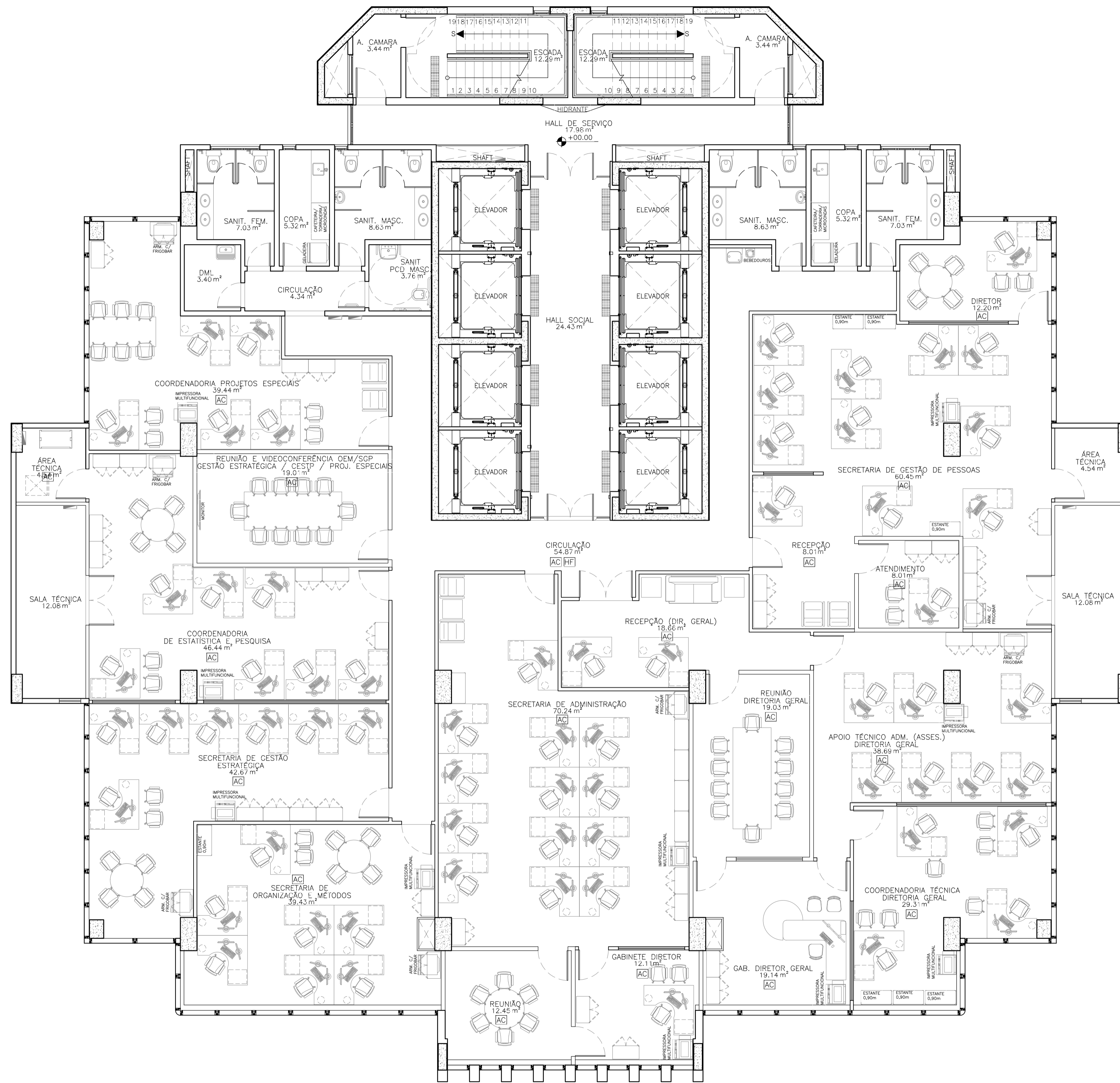
01 PLANTA LAYOUT – 8º PAV. ESCALA: 1/75
