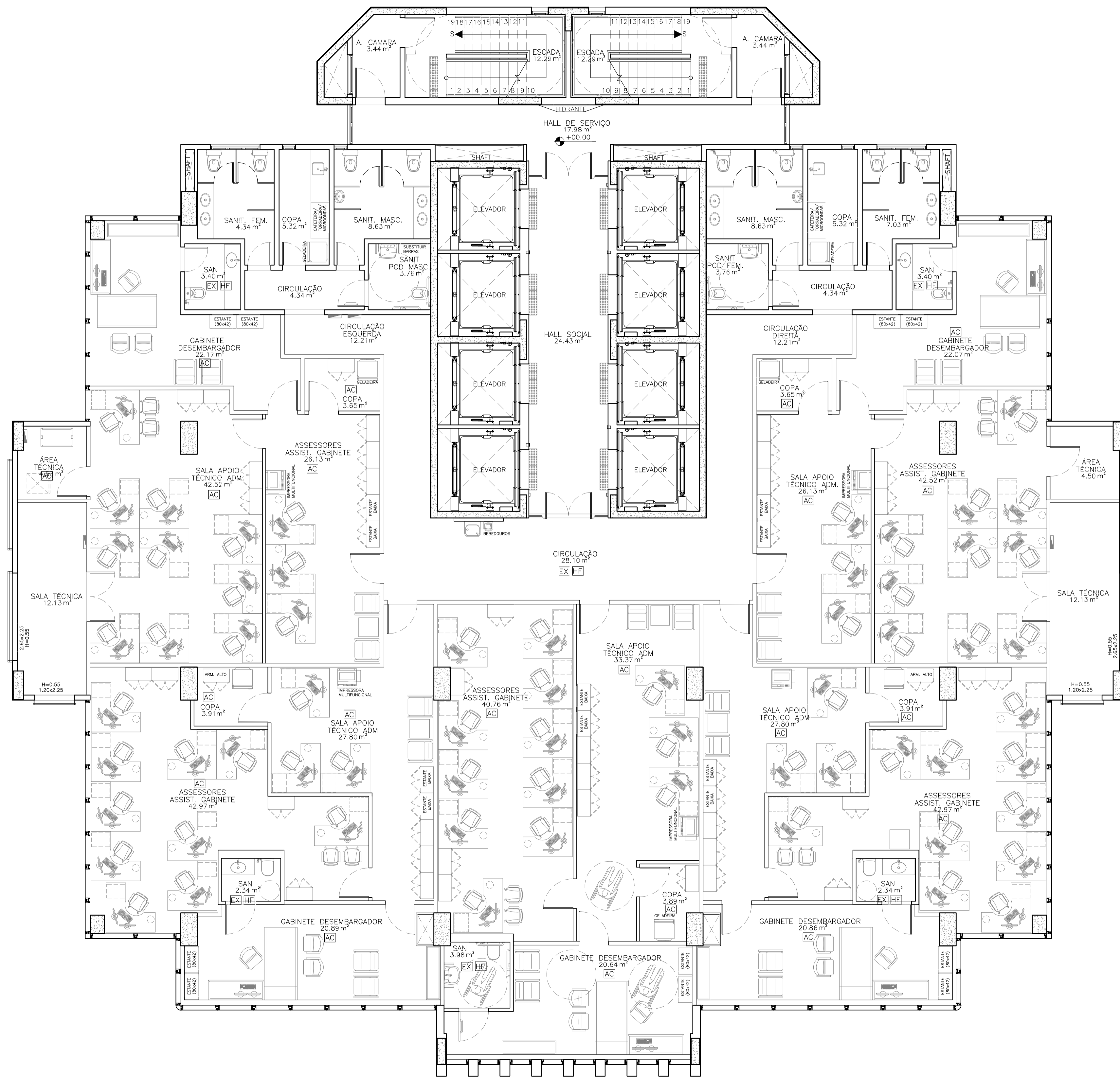
01 PLANTA LAYOUT - 13° AO 15° PAV. ESCALA: 1/75
